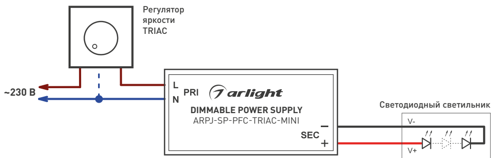
Рис. 1. Подключение драйвера.
