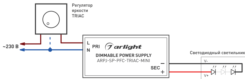
Рис. 1. Подключение драйвера.
