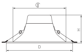
Рис. 1. Чертеж и габаритные размеры
