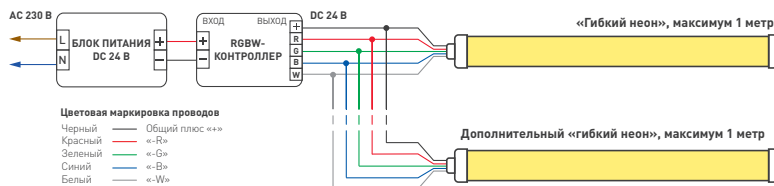
Схема 1. Подключение «гибкого неона» с использованием 4-канального RGBW-контроллера с возможностью изменения цвета свечения и яркости
